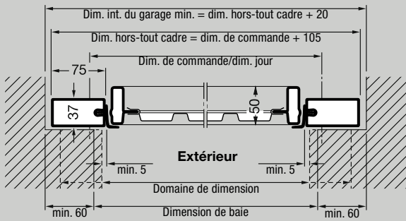
Coupe horizontale
